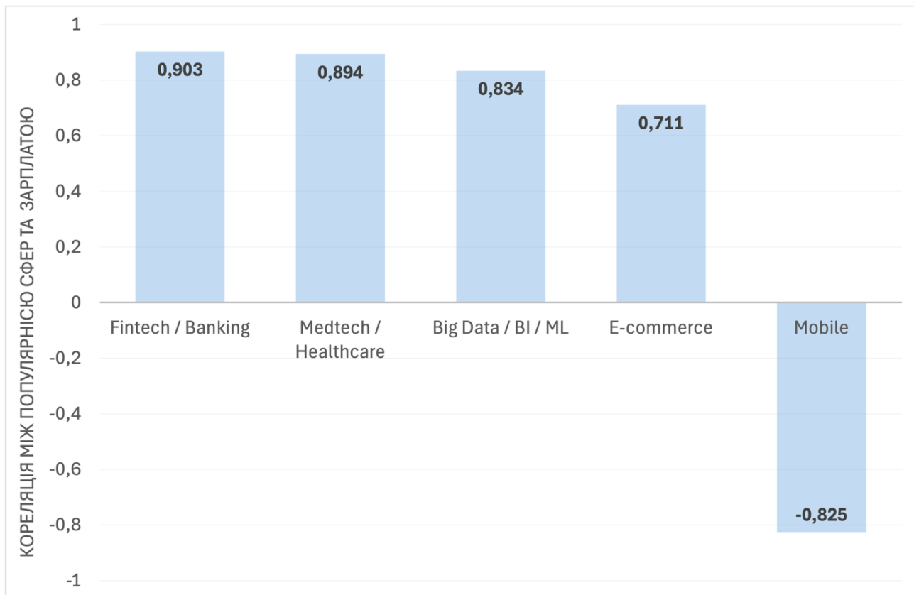
Рис. 2. Кореляція Пірсона між популярністю сфер та середньою зарплатою, 2014-2023 роки
